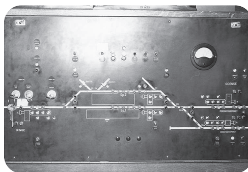
Da stationen havde fået nyt relæsikringsanlæg, kunne sporskifter og signaler betjenes fra denne sportavle placeret på stationskontoret. Foto: Ole Edvard Mogensen/Dalum-Hjallese Lokalarkiv
